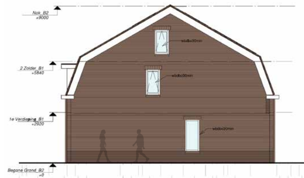
WESTGEVEL
