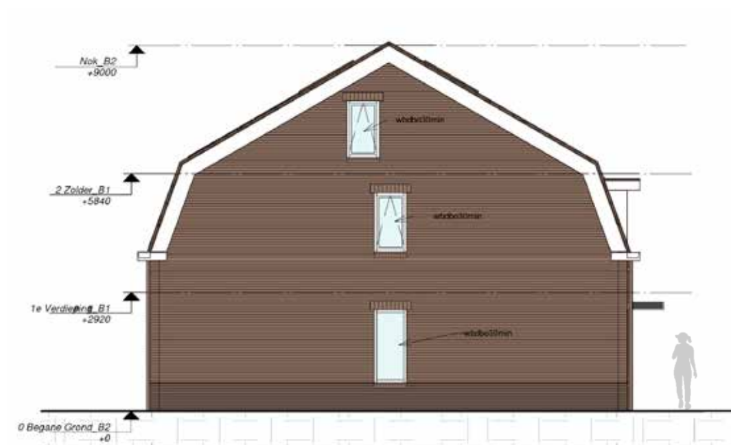
OOSTGEVEL
